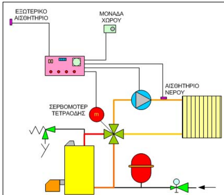
Εικόνα 3.2.5. Τυπική διάταξη αντιστάθμισης σε εγκατάσταση θέρμανσης με τετράοδη βάνα αναμείξεως
