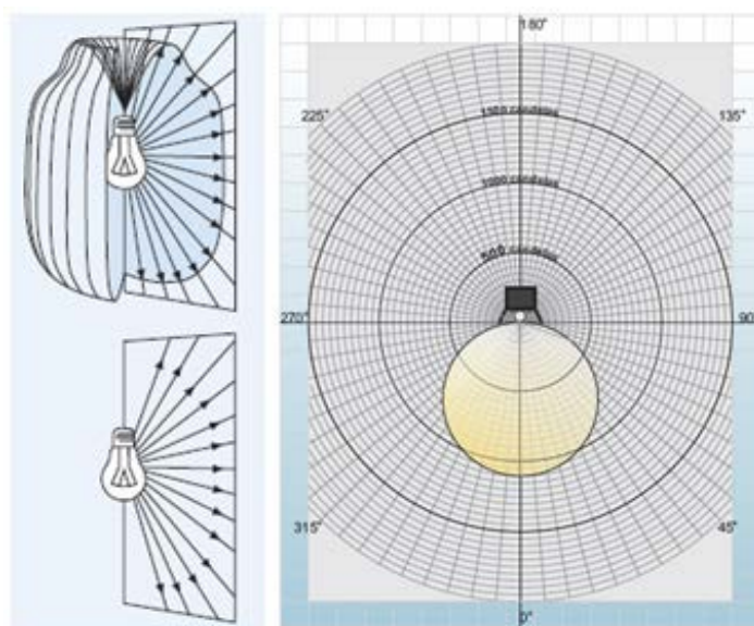
Σχήμα 1.4.4 Πολική κατανομή φωτεινής έντασης.
