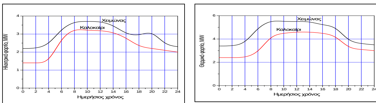
Σχήμα 2.7.2. Παράδειγμα ωριαίου ημερήσιου προφίλ ηλεκτρικού και θερμικού φορτίου
