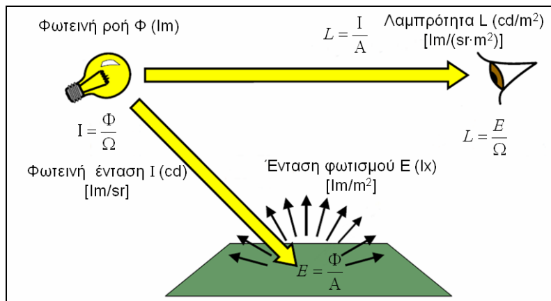
Σχήμα 1.4.5 Συσχέτιση μεταξύ των βασικών φωτομετρικών μεγεθών.
