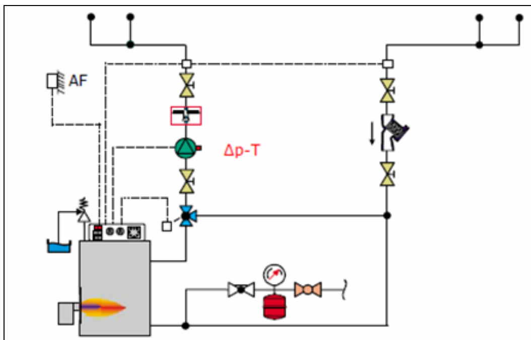
Σχήμα 1.4. Σύστημα αντιστάθμισης σε εγκατάσταση θέρμανσης με τρίοδη βάνα αναμειξεως.
