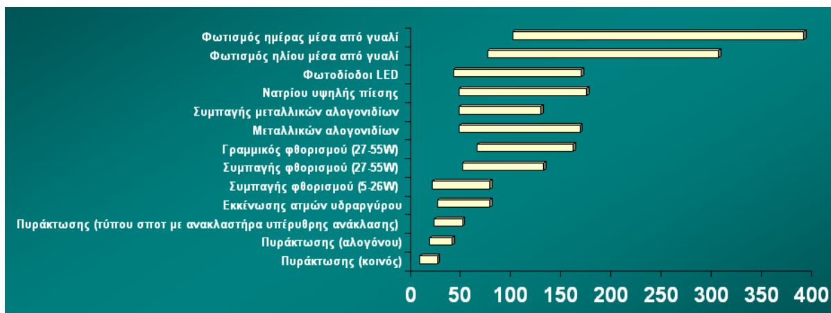
Σχήμα 1.4.6 Απόδοση λαμπτήρων σε lm/W συμπεριλαμβανομένου του συστήματος έναυσης και λειτουργίας όπου αυτό απαιτείται.
