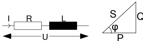
Σχήμα 3.2.15. R - L φορτίο και διάγραμμα ισχύος
