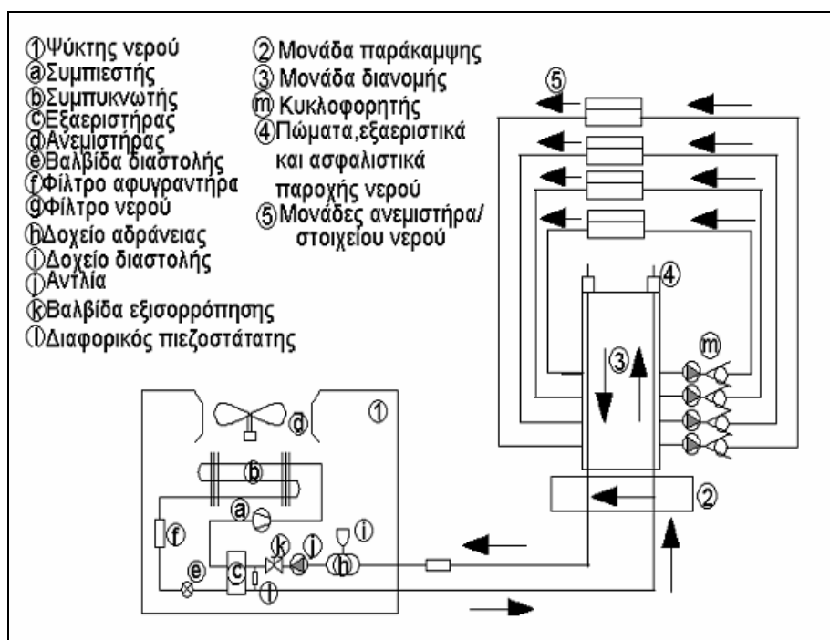
Σχήμα 2.3.3 Συγκρότηση πολυζωνικού συστήματος νερού
