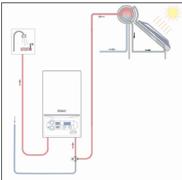
Εικόνα 2.11.3. Σχηματική απεικόνιση επιτοίχιου λέβητα αερίου συμπτκνώσεως, όπου λειτουργεί ως ταχυθερμαντήρας, αλλά και ως μεταθερμαντής του ζεστού νερού από τον ηλιακό θερμοσίφωνα
